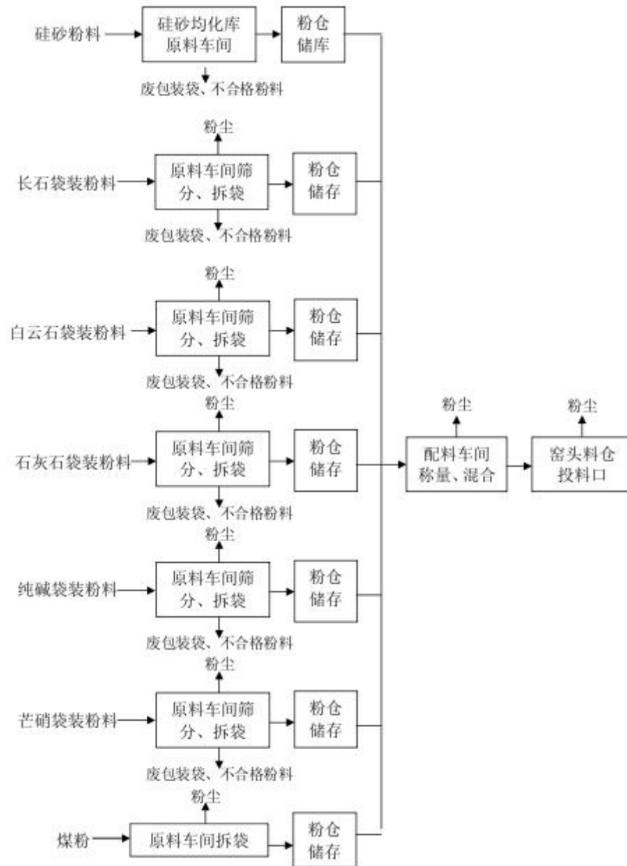
图 3.1-3 原料车间工艺流程及产污节点图
