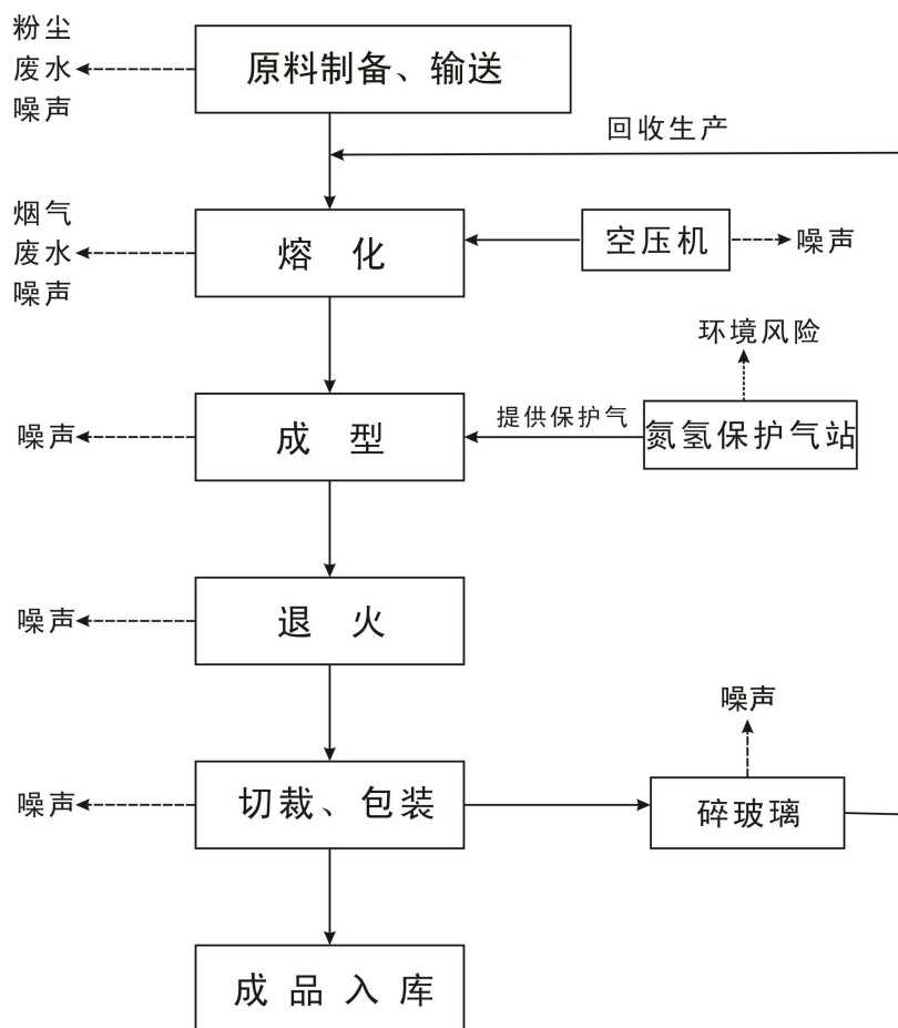
图 3.1-1 浮法玻璃生产线工艺流程及产污节点
