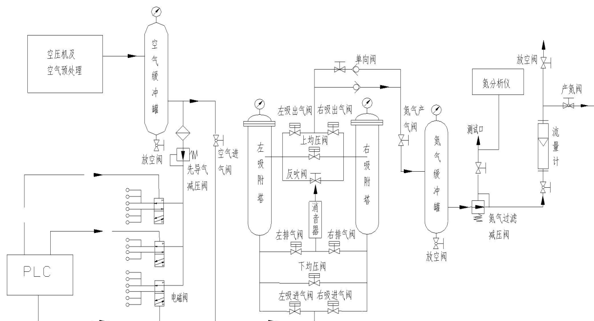
图 3.1-4 PSA 空分制氮工艺流程图
