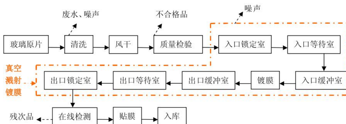
图 3.1-2 低辐射镀膜节能玻璃生产线工艺流程及产污节点图
